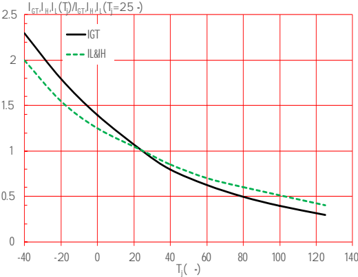
FIG.7: I_{GT}/I_{GT}(T)/I_{GT}(T=25^\circ C) I_{L&H}/I_{L&H}(T)/I_{L&H}(T=25^\circ C)
